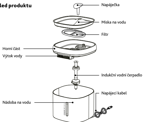
Indukční vodní čerpadlo
