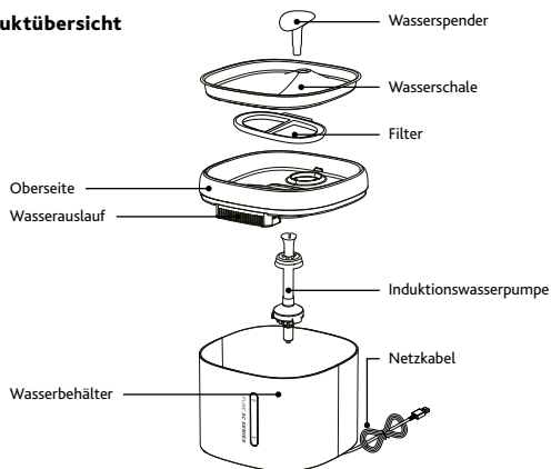
Induktionswasserpumpe
